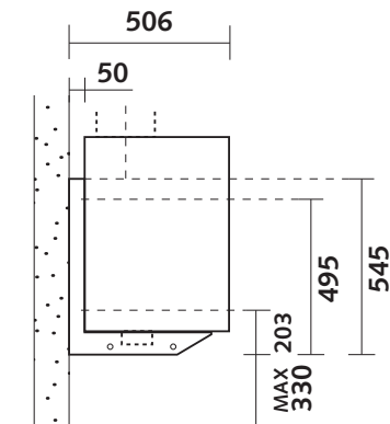
SEITENANSICHT
