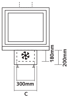
VOORAANZICHT
