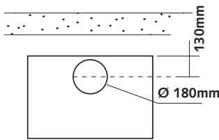
BOVENAANZICHT
