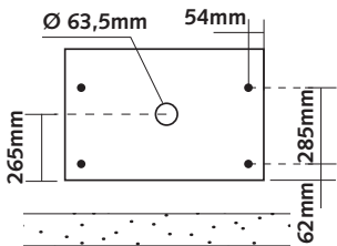
ONDERAANZICHT
