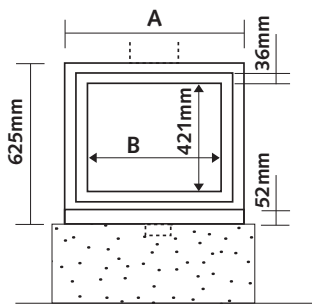
VOORAANZICHT
