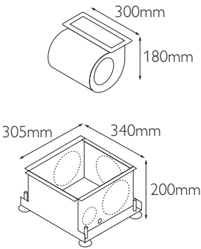
S16-CUBE 58 KIT DE VENTILATION (VENTILATEUR + CAISSON)
