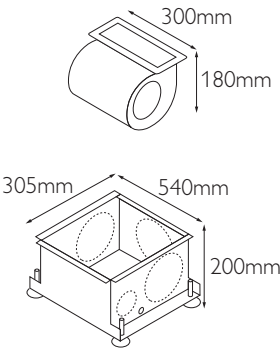
S16-CUBE 68 & S16-CUBE 78 KIT DE VENTILATION (VENTILATEUR + CAISSON)
