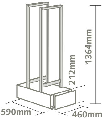
S16-CUBE 68 & S16-CUBE 78 KIT DE VENTILATION (VENTILATEUR + CAISSON)
