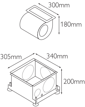
S16-CUBE 58 JUEGO DE VENTILACIÓN (VENTILADOR + CAJA)
