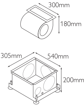
S16-CUBE 68 Y S16-CUBE 78 JUEGO DE VENTILACIÓN (VENTILADOR + CAJA)
