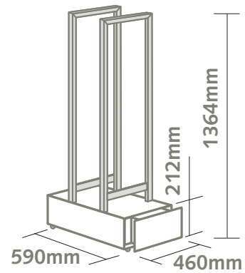
S16-CUBE 68 & S16-CUBE 78 VENTILATOR-BAUSATZ (VENTILATOR + VENTILATIONSKASTEN)
