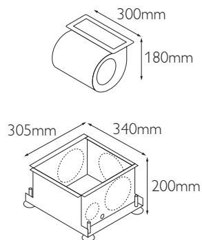
S16-CUBE 58 VENTILATOR-BAUSATZ (VENTILATOR + VENTILATIONSKASTEN)
