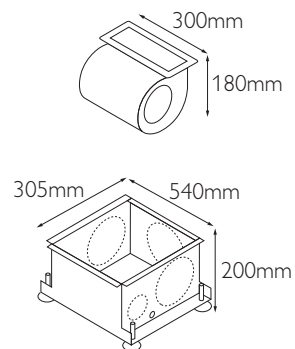
S16-CUBE 68 & S16-CUBE 78 VENTILATOR-BAUSATZ (VENTILATOR + VENTILATIONSKASTEN)
